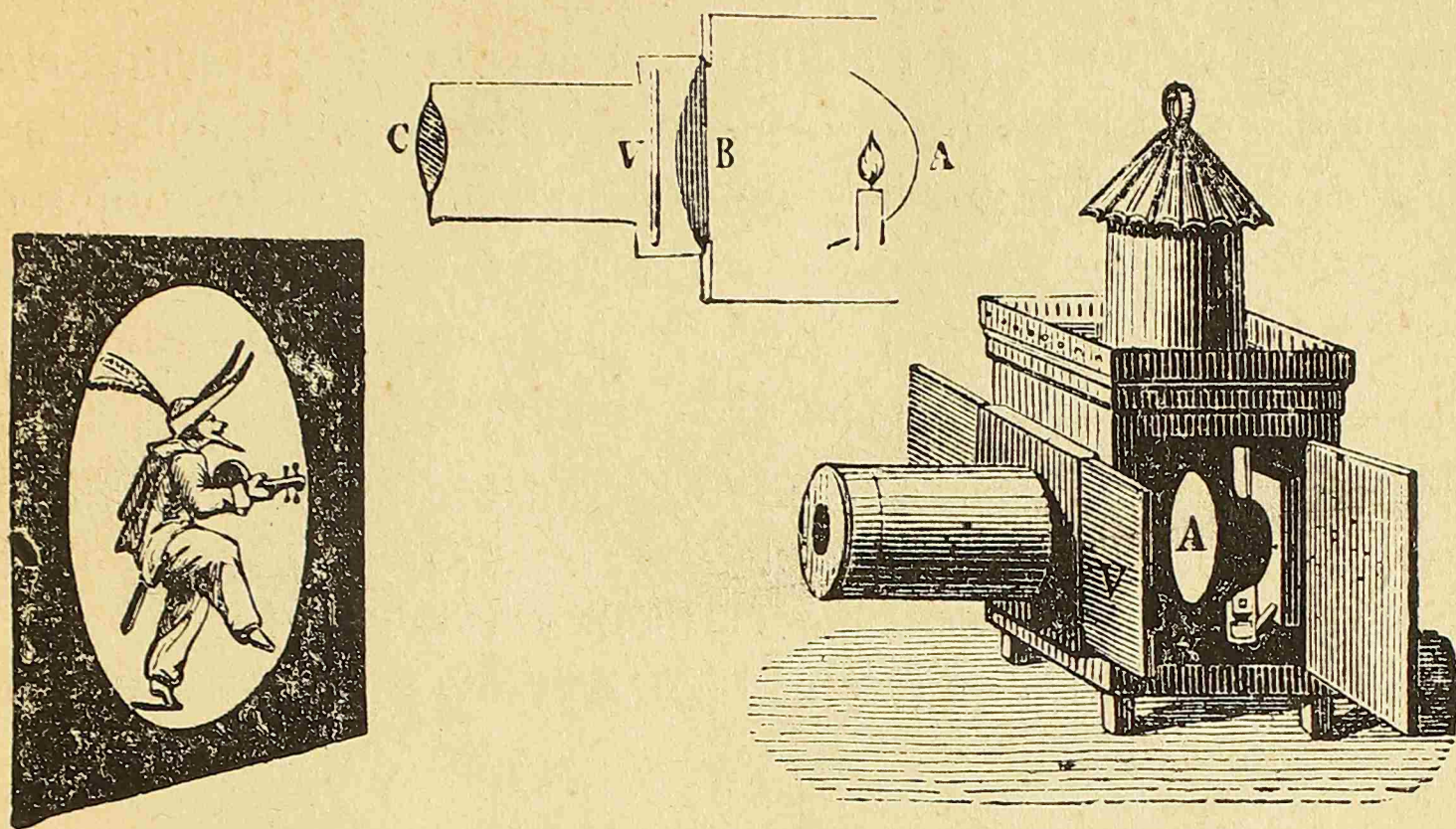
Fig. 17. — Linterna mágica.
