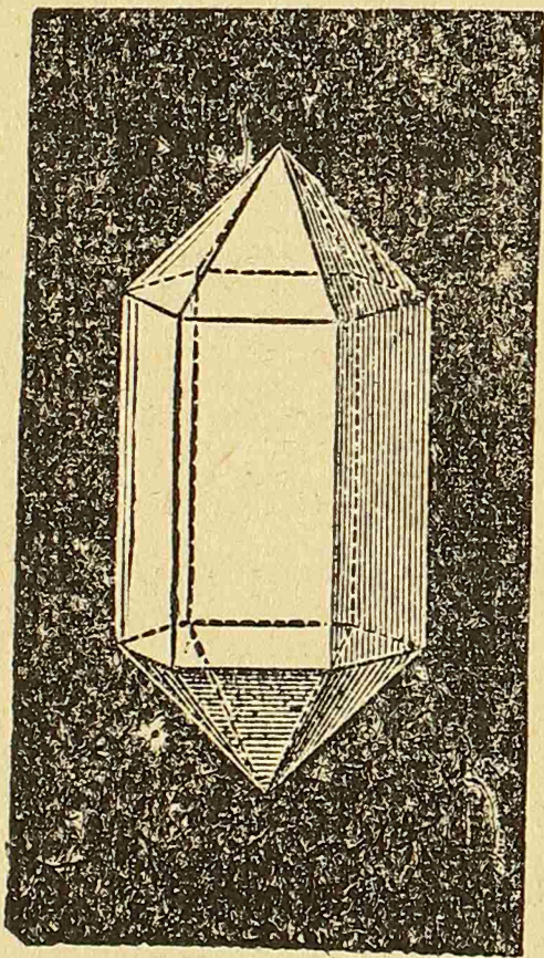
Fig. 25. — Cristales de roca.
