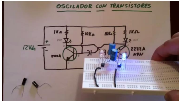
Circuito oscilador: de la teoría a la práctica (Tecnología)
