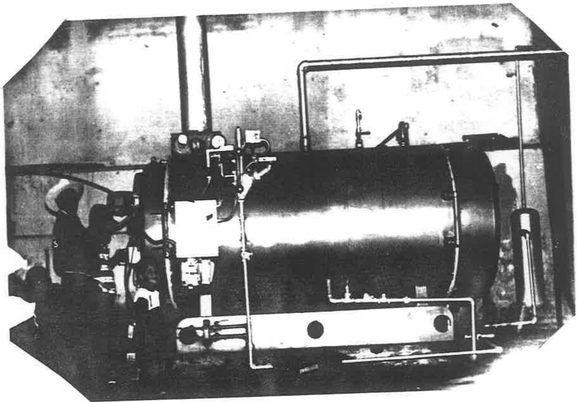
17.- Caldera generadora de vapor para el proceso
